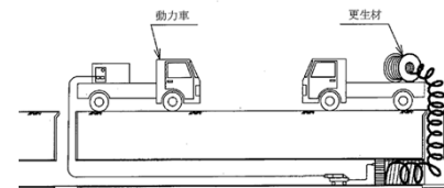
管更生(製管工法)
