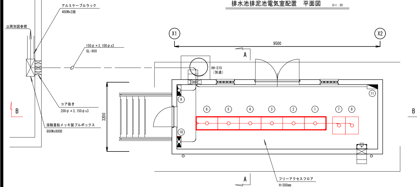
排水池排泥池電気室配置 平面図 S=1:50
