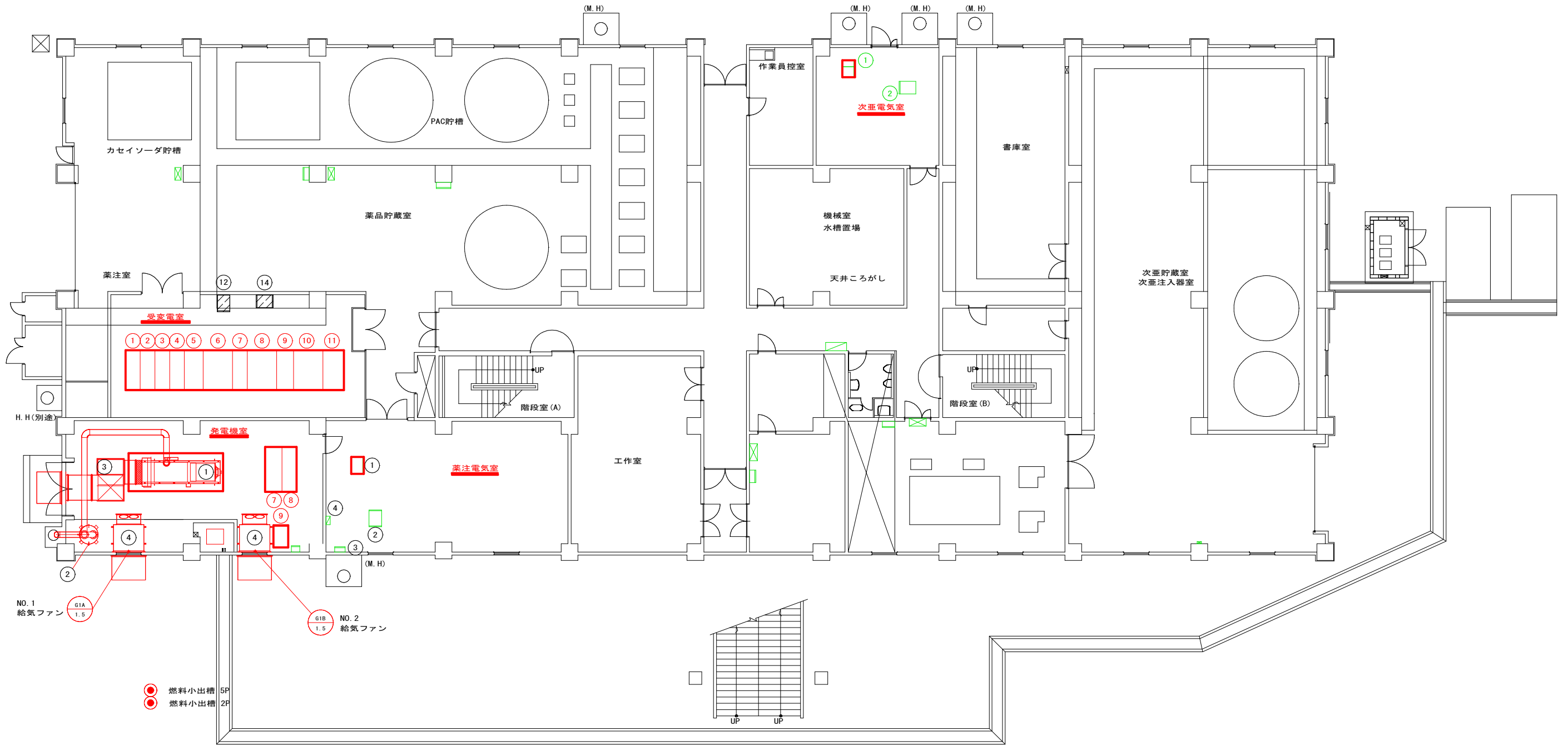
管理本館1階 平面図 1/100
