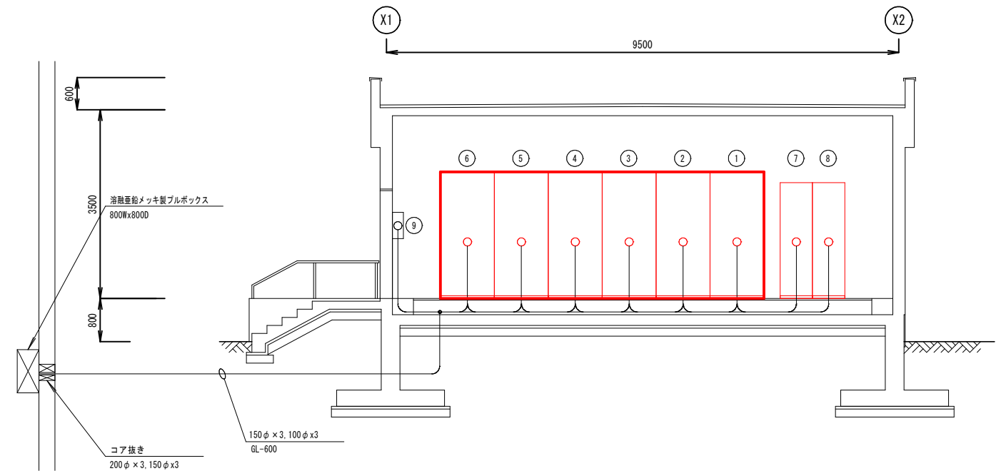
B-B 断面图 S=1:50
