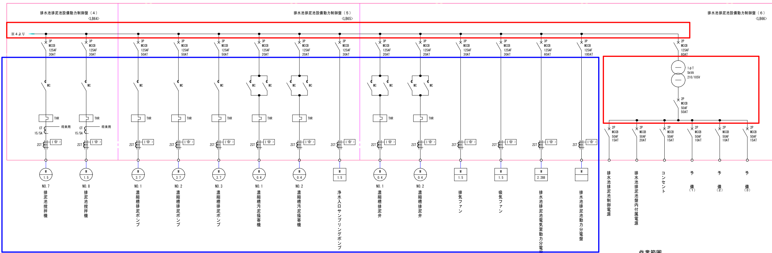
排水池排泥池設備動力制御盤単線結線図
