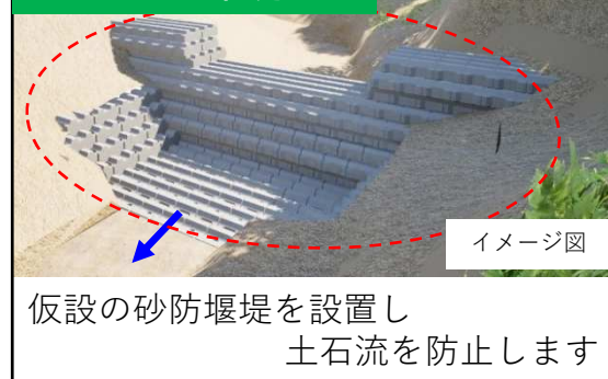
ブロック堰堤工
