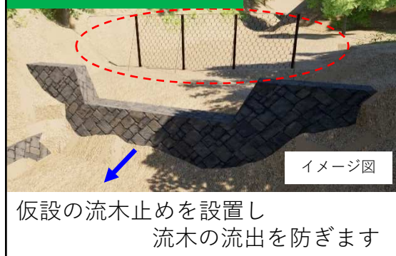
強靱ワイヤーネット工
