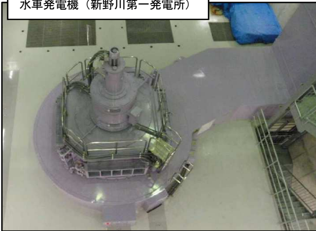
水車発電機（新野川第一発電所）
