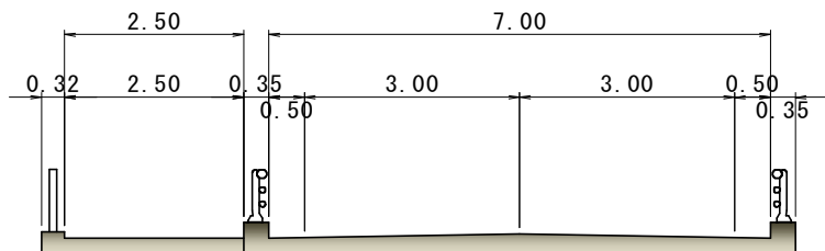
現況横断図(橋梁部)
