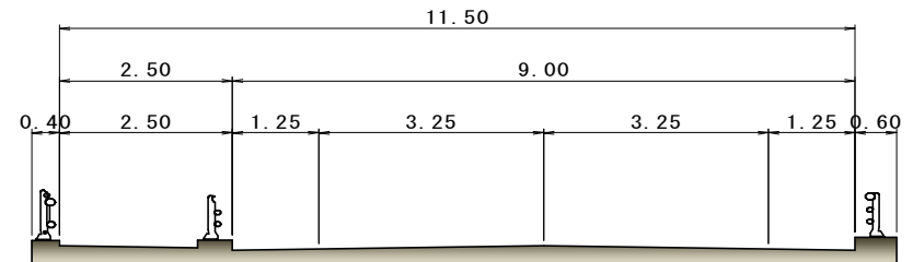
計画横断図(橋梁部)
