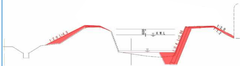
計画断面図
