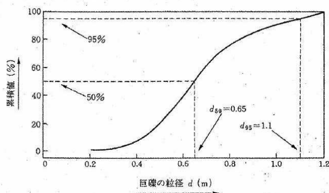
図－2 巨礫の粒径の累加曲線例
