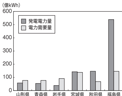
東北6県の発電電力量・需要量 （令和5年度）
